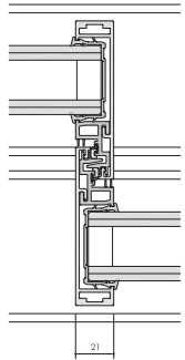
Detail van middenstijl
