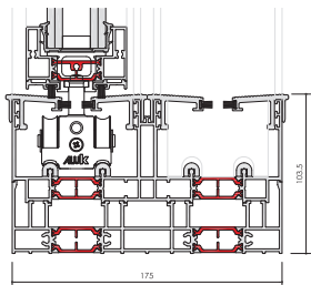
Onderste deel van de configuratie van een vlakke dorpel
