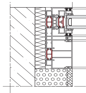
Detail van stijl
